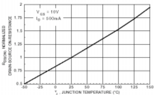
图 3. 导通电阻-结温
