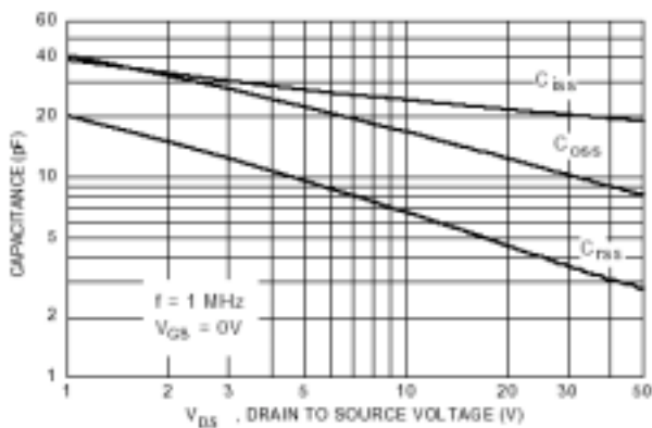
图 9. 电容特性
