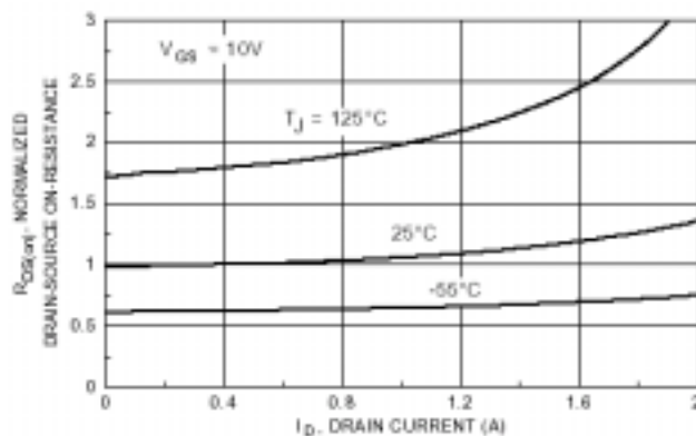
图 4. 导通电阻-漏极电流、结温
