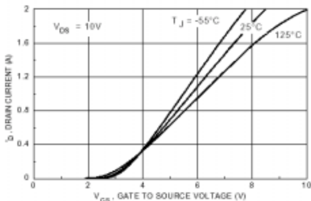
图 5. 转移特性
