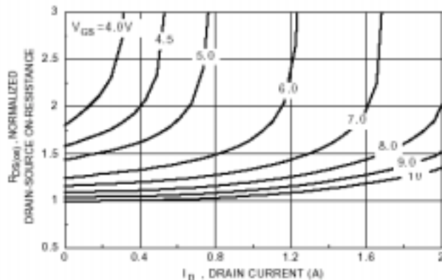
图 2. 导通电阻-栅极电压、漏极电流
