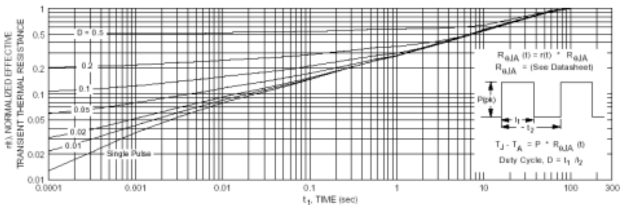
图 14. 瞬态热阻
