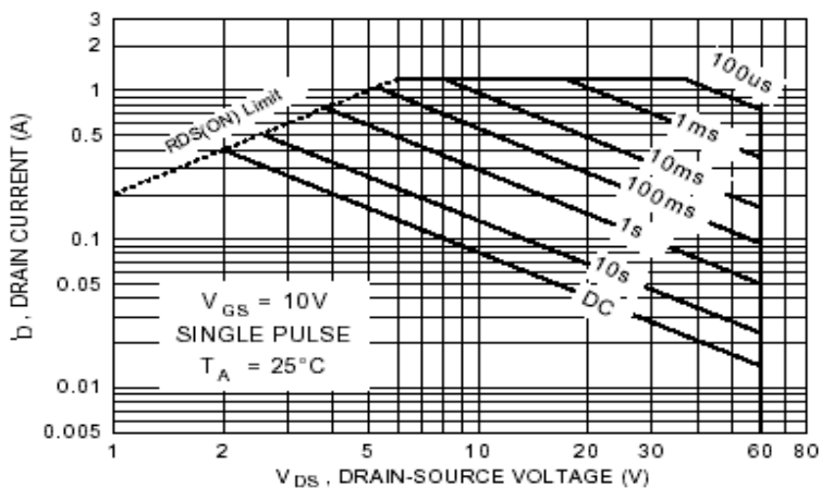
图 13. 最大安全工作区
