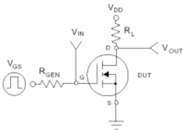
图 11. 开关时间测试电路
