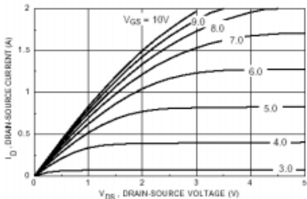
图 1. 导通特性
